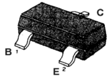
SOT-23
